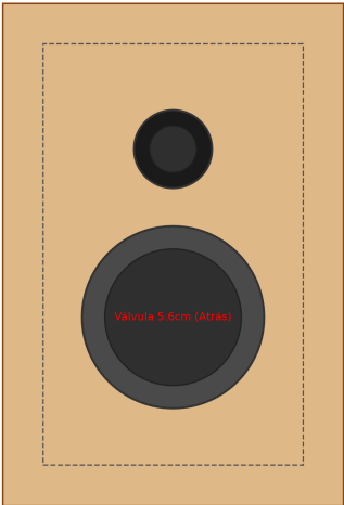
Caja Izquierda (L)
